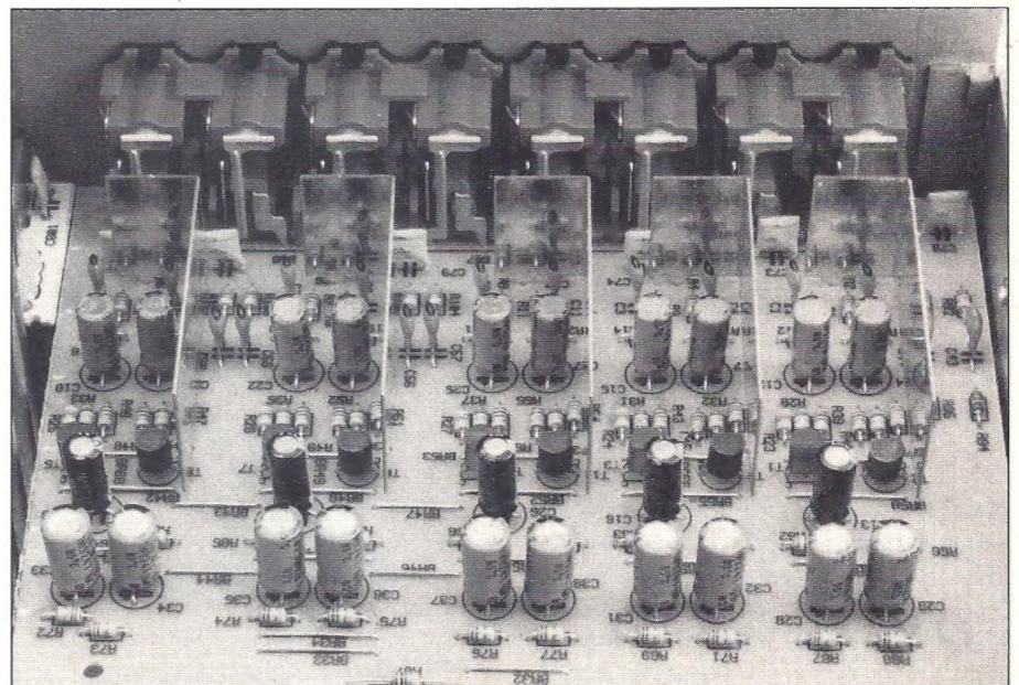
Detailopname van de opbouw van de ingangskonfiguratie. Bijzonder netjes zijn de afscherm-schotjes, waardoor overspraak vermeden wordt.
